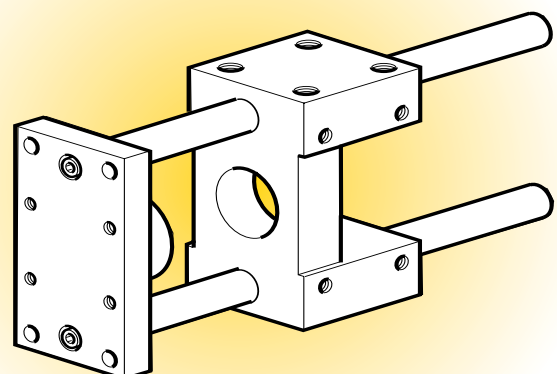
Parallelführung (Verdrehsicherung)
