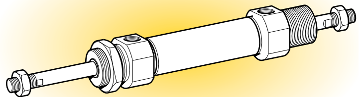
Doppeltwirkend, durchgehende Kolbenstange
